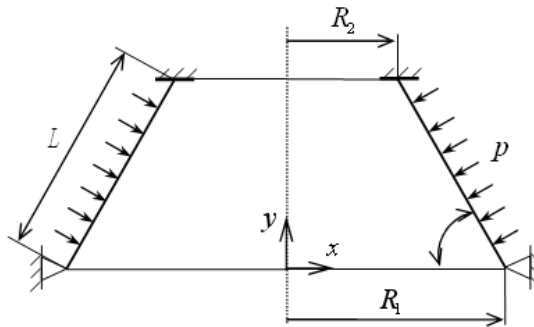
Рисунок 2. Геометрия оболочки
